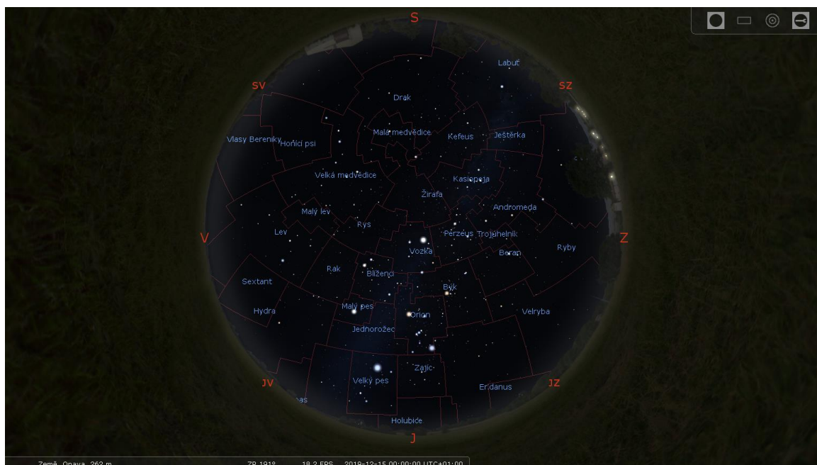
Obrázek 53: Hvězdná obloha v ČR 15. prosince v 00.00 hodin SEČ 51
